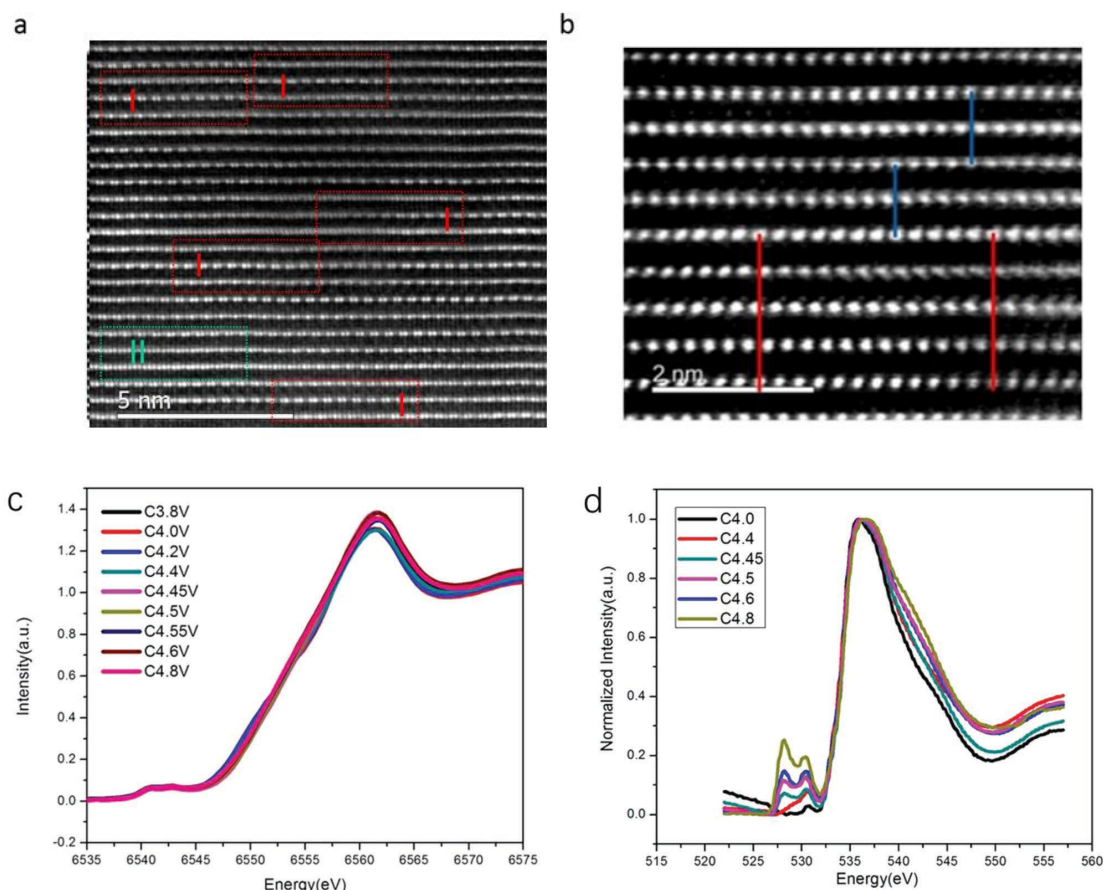
a) \text{Li}_{1.25}\text{Co}_{0.25}\text{Mn}_{0.5}\text{O}_2 样品的高角环形暗场 (HAADF) 图像; b) 基于 P6_3mc 空间群, 沿 100 方向放大 HAADF 图像; c) 不同充电电压下, 归一化的锰 K 边 X 射线吸收谱; d) 不同充电电压下, 氧 K 边软 X 射线吸收谱。
