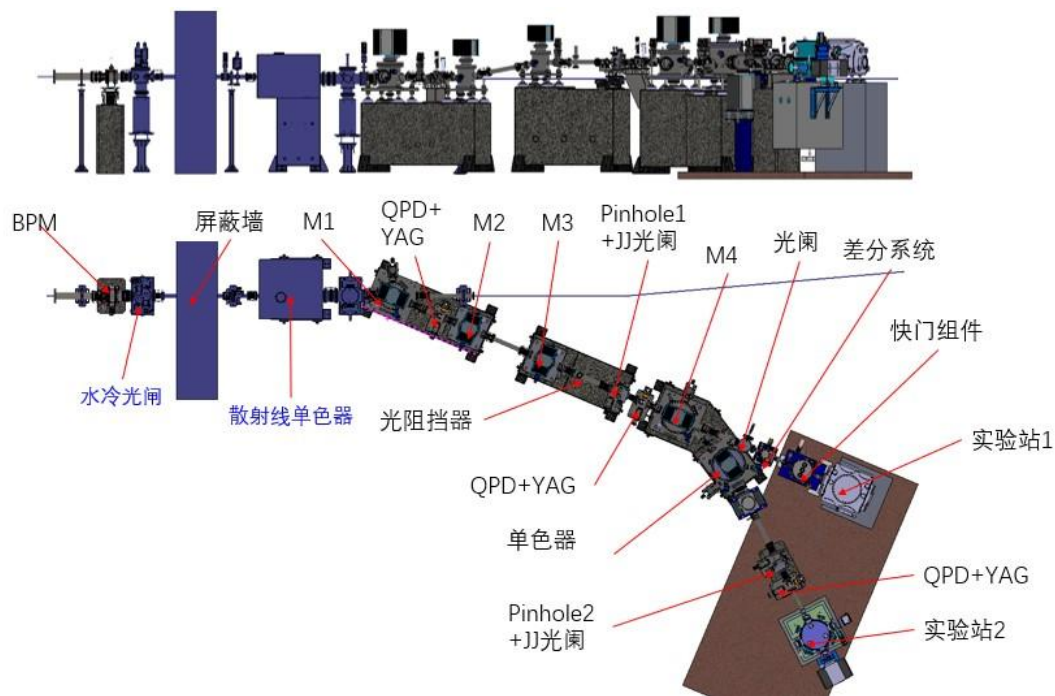
图 3.1-7 金华光束线散射线及支线示意图
