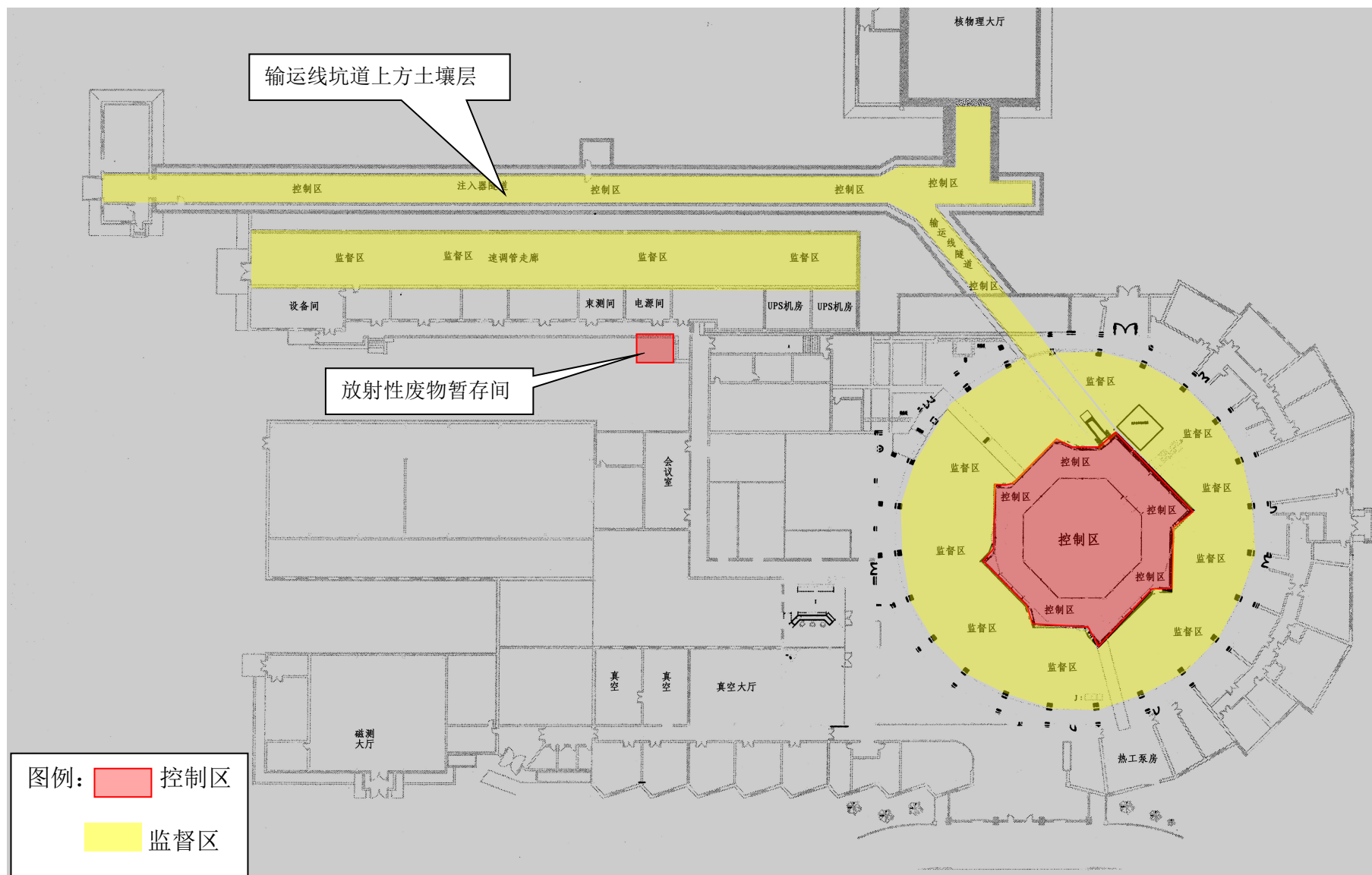
图 4.1-1 (b) 合肥光源辐射工作场所分区图 (地上部分)
