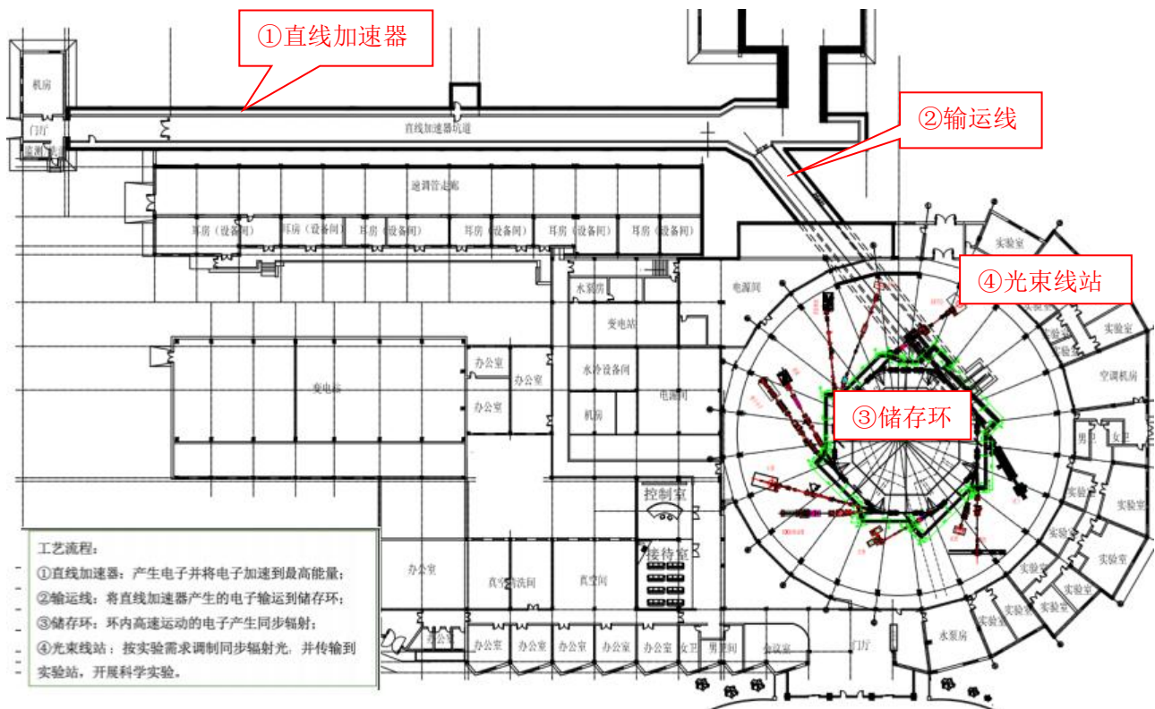
图3.2-4 HLS装置工艺流程图
