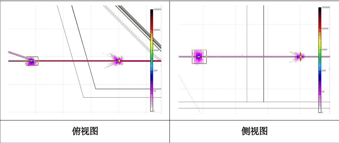
图 5.2-25 支线气体轫致辐射计算结果
