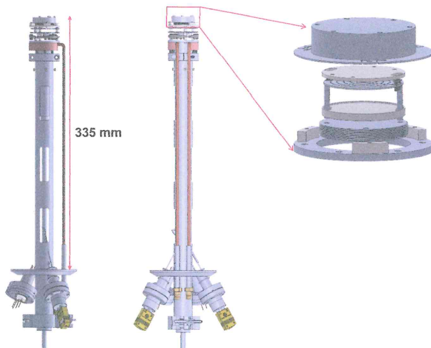
附件：电阻激光复合加热样品架的结构示意图
