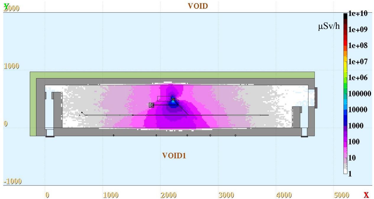
图 5.2-6(a) 调试模式 3 下加速器测试大厅束流平面（标高 0.1m）的剂量率水平分布
