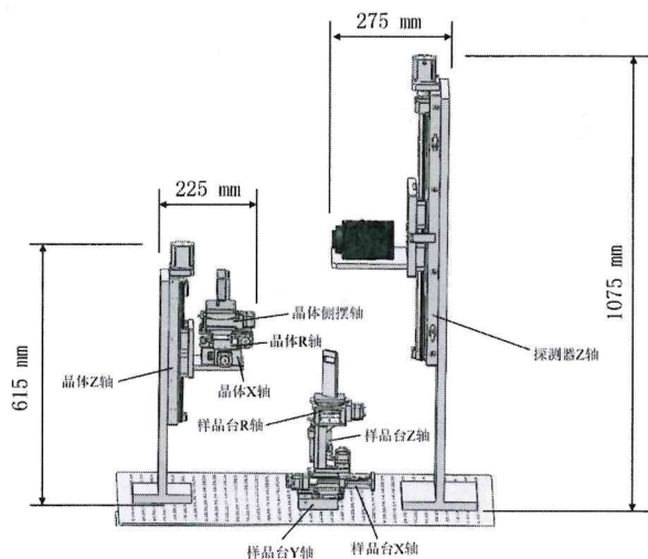
图 1 光谱仪真空运动机构示意图
